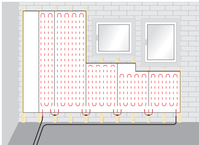
Abb. 217 Flexible Montagemöglichkeiten zur Anpassung an bauliche Gegebenheiten
