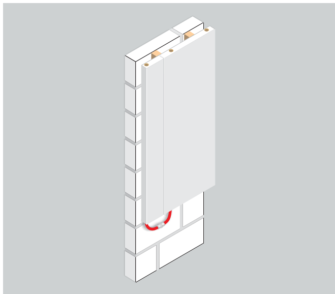
Abb. 216 Wandaufbau Fonterra Side 12
