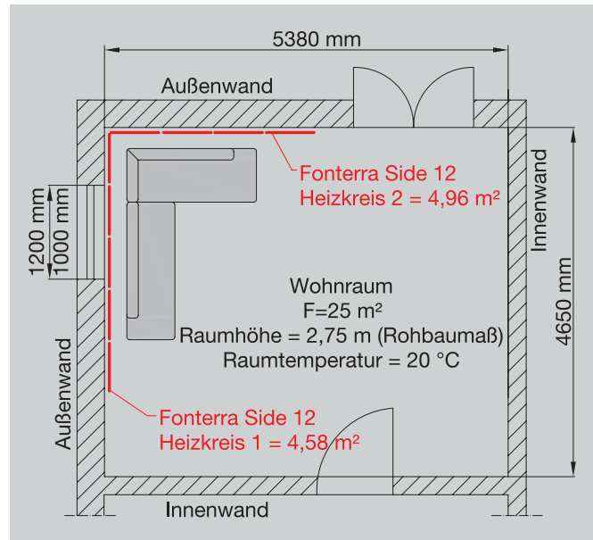
Abb. 219 Mögliche Anordnung der benötigten Wandheizplatten
