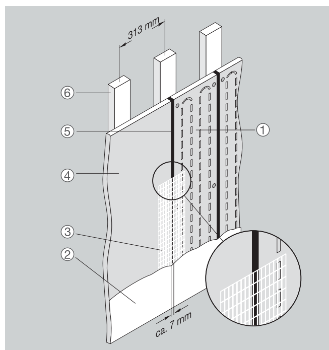
Abb. 224 Anschluss Wandheizplatte an Gipskartonplatte (inaktive Fläche)
