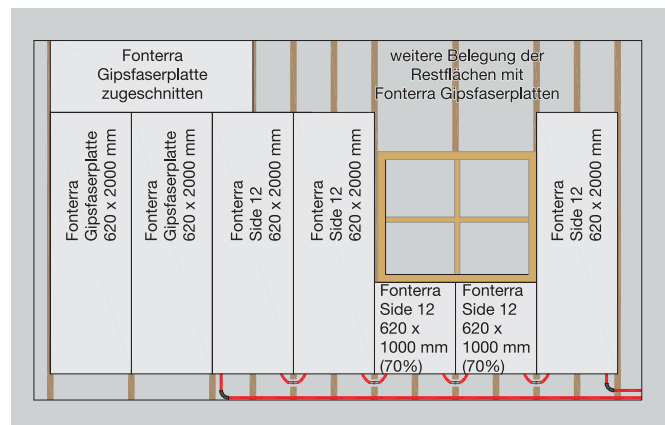
Abb. 220 Wandansicht Musterraum mit möglicher Systemplattenanordnung
